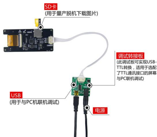
图 1-3 调试工具图
