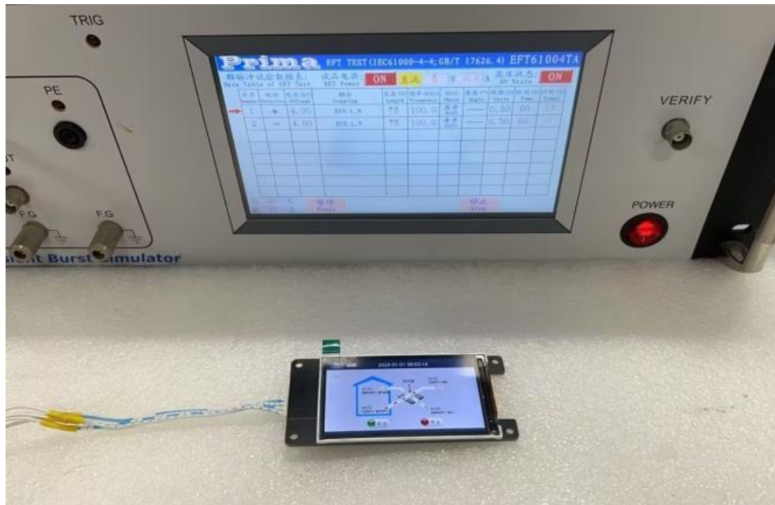
图 4-3 EFT 测试图
